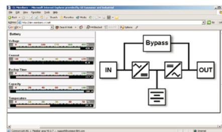
USV Datenwerte
